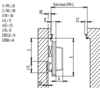
Ingombri massimi Unirev REI 60 / REI 120
