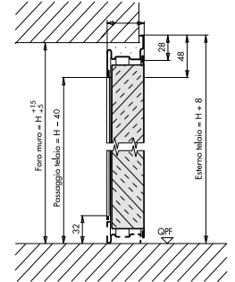
Sezione verticale Unirev multiuso
