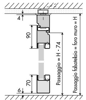
Sezione verticale Vetrac REI 30 / REI 60
