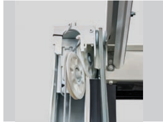
La dimensione delle carrucole di rinvio garantisce lunga durata alla fune in acciaio e un corretto posizionamento del contrappeso.
